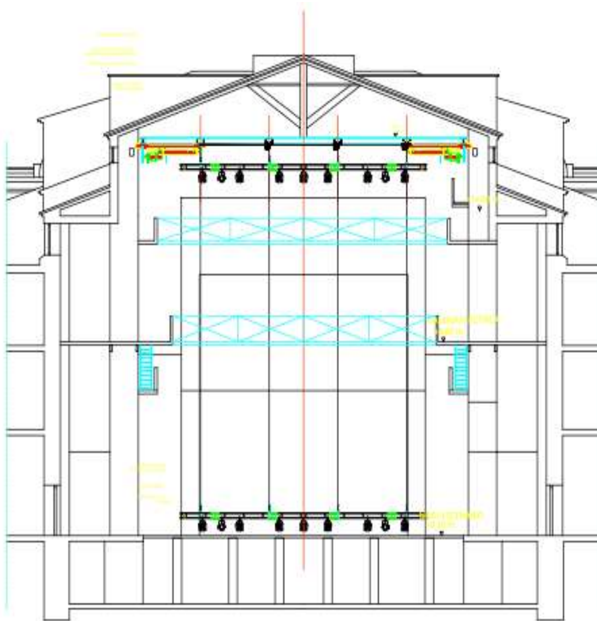
SECCION TRANSVERSAL
